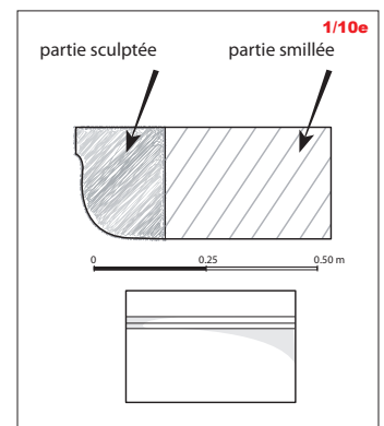
Bloc architectural (corbeau)
