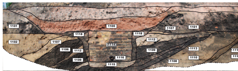
Coupe stratigraphique d'un aménagement ferroviaire du XXe siècle réalisé au sein d'une levée de terre massive effectuée vers le milieu du XIXe siècle
